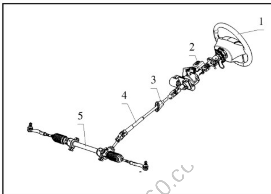
(1) 转向盘总成 (2) 转向管柱 (3) 转向防尘罩 (4) 转向下传动轴 (5) 转向器总成
